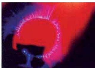
Obr. č. 9 Nativní snímek elektrografie – vysokofrekvenční korónový výboj na prstu probanda
